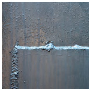
Schweißverbindung
